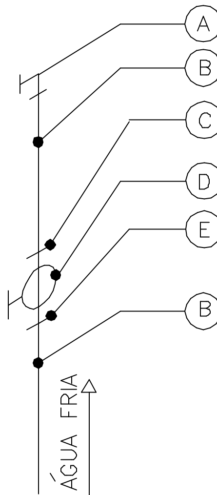
DETALHE DE INSTALAÇÃO DE CHUVEIRO COM ÁGUA FRIA
