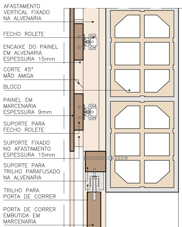
DETALHE - PAINEL ACABAMENTO ESC. 1:5
