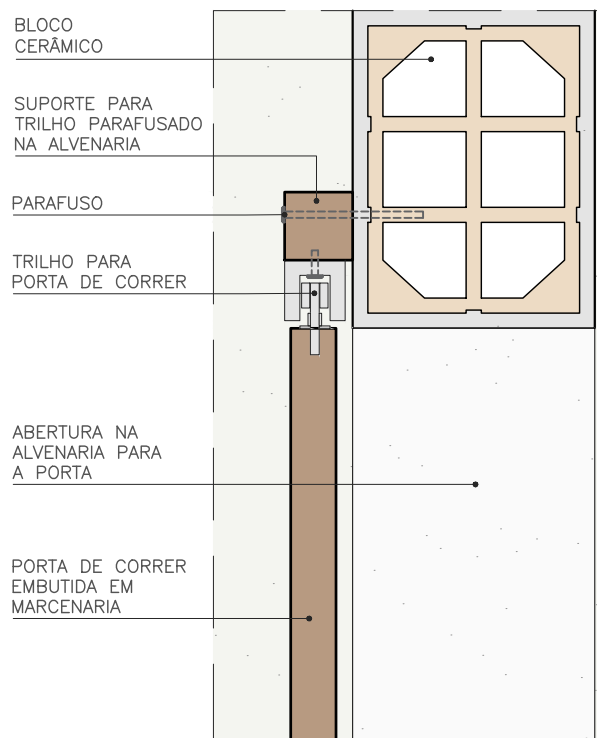
DETALHE - PORTA E TRILHO ESC. 1:5
