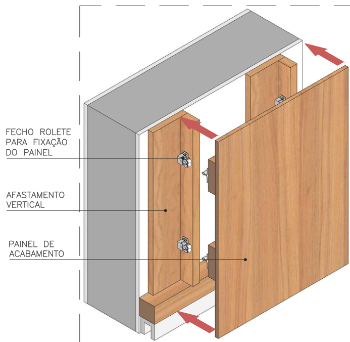
ISOMÉTRICA - PAINEL ACABAMENTO SEM ESCALA
