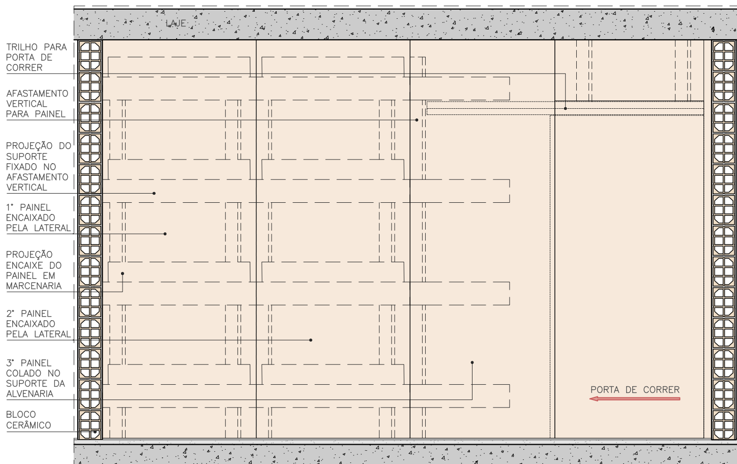
VISTA FRONTAL ESC. 1:25
