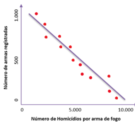
Correlação Negativa
