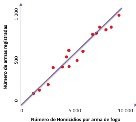
Correlação Positiva
