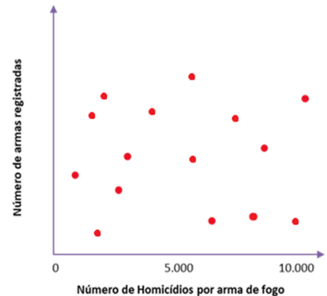
Nenhuma Correlação
