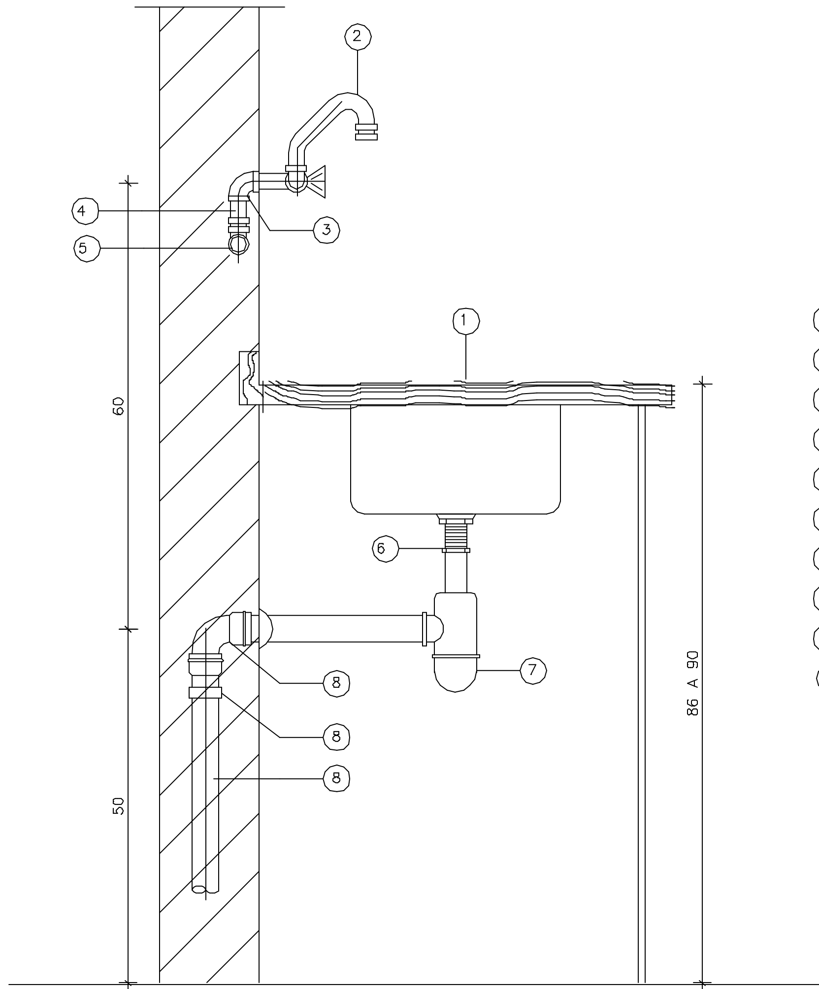
DETALHE DE INSTALAÇÃO DA PIA
