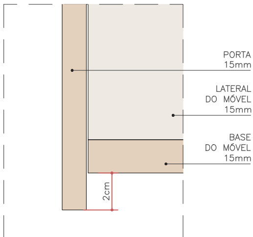
SUPERIORES ESC. 1:2
