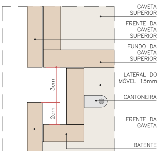
GAVETEIRO ESC. 1:2
