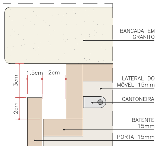
INFERIORES ESC. 1:2
