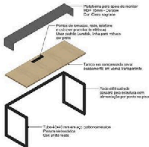
1 Det. Mesa ADM A303 1:25
