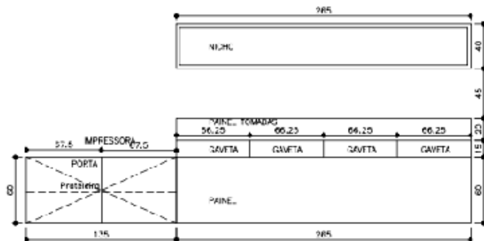
ELEVAÇÃO ESCRITÓRIO
