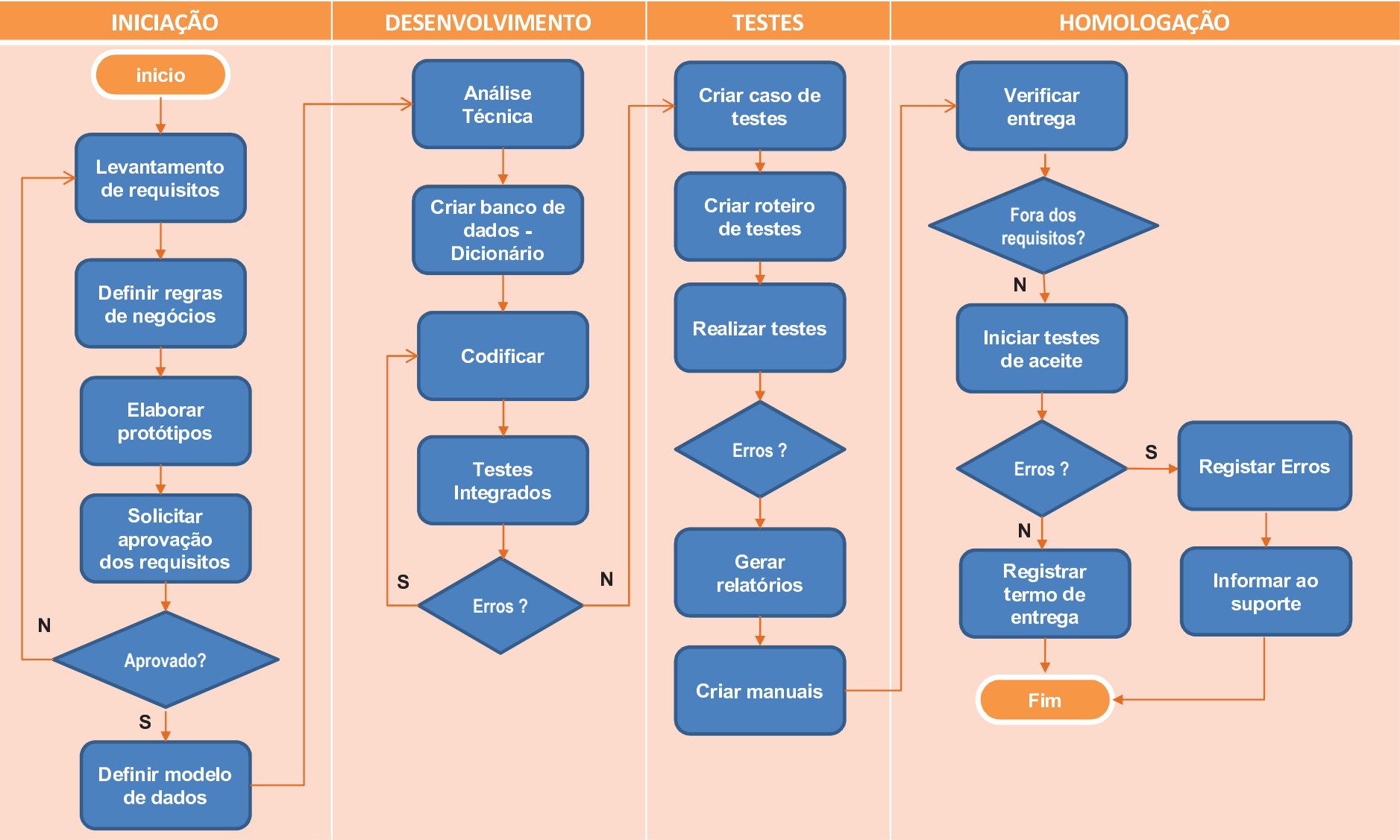
Detalhamento do fluxograma ligando artefatos do MDS
