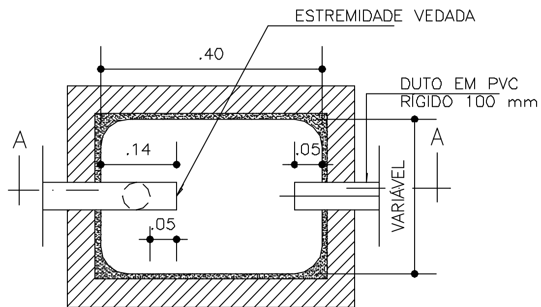
PLANTA BAIXA
