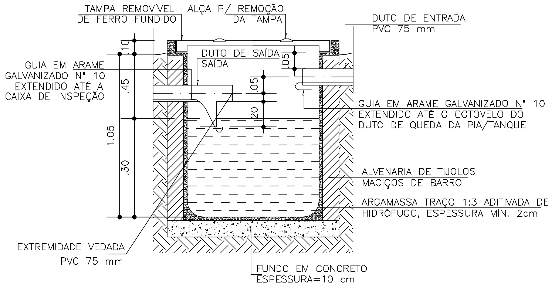
CORTE AA
