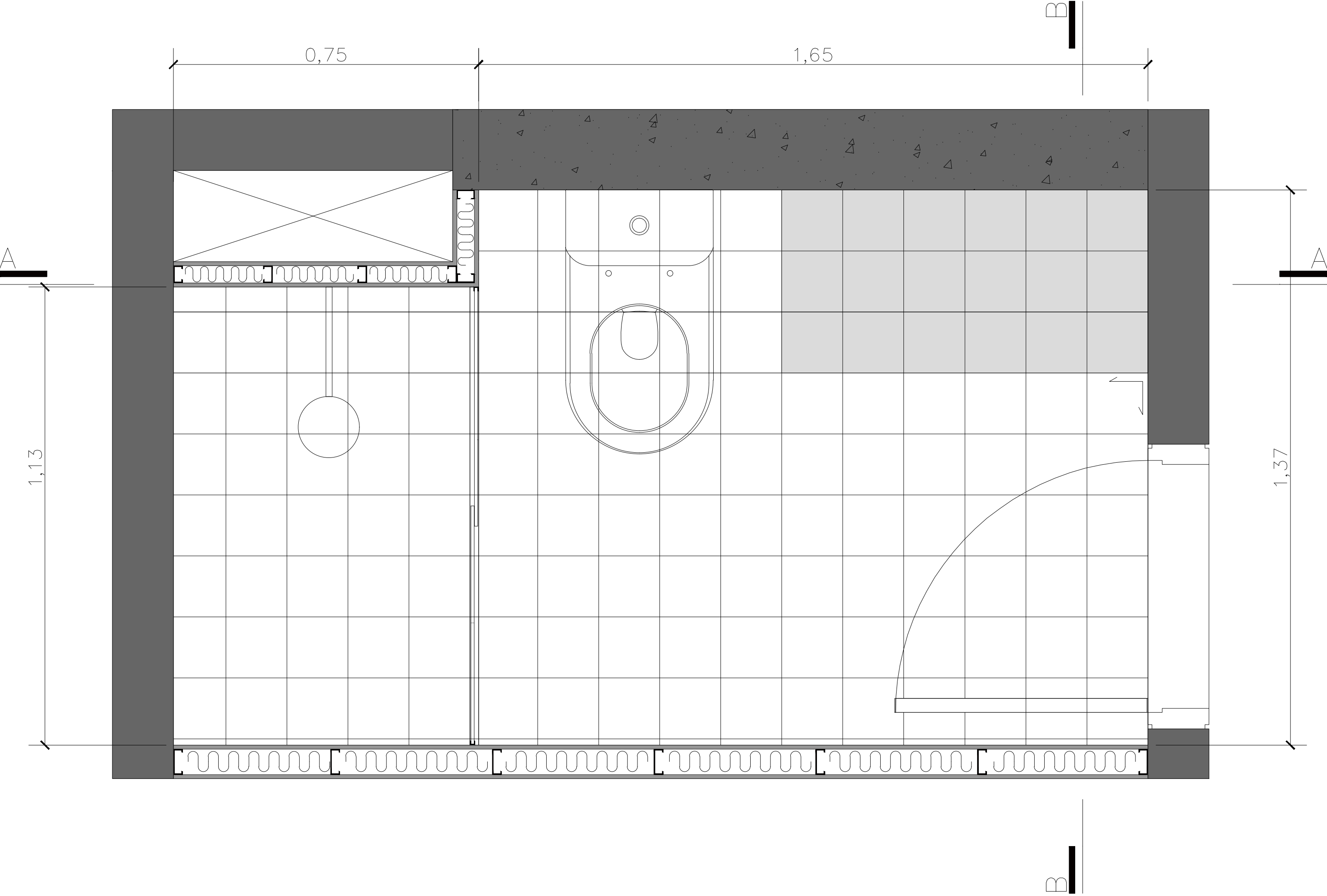
Planta Banheiro
