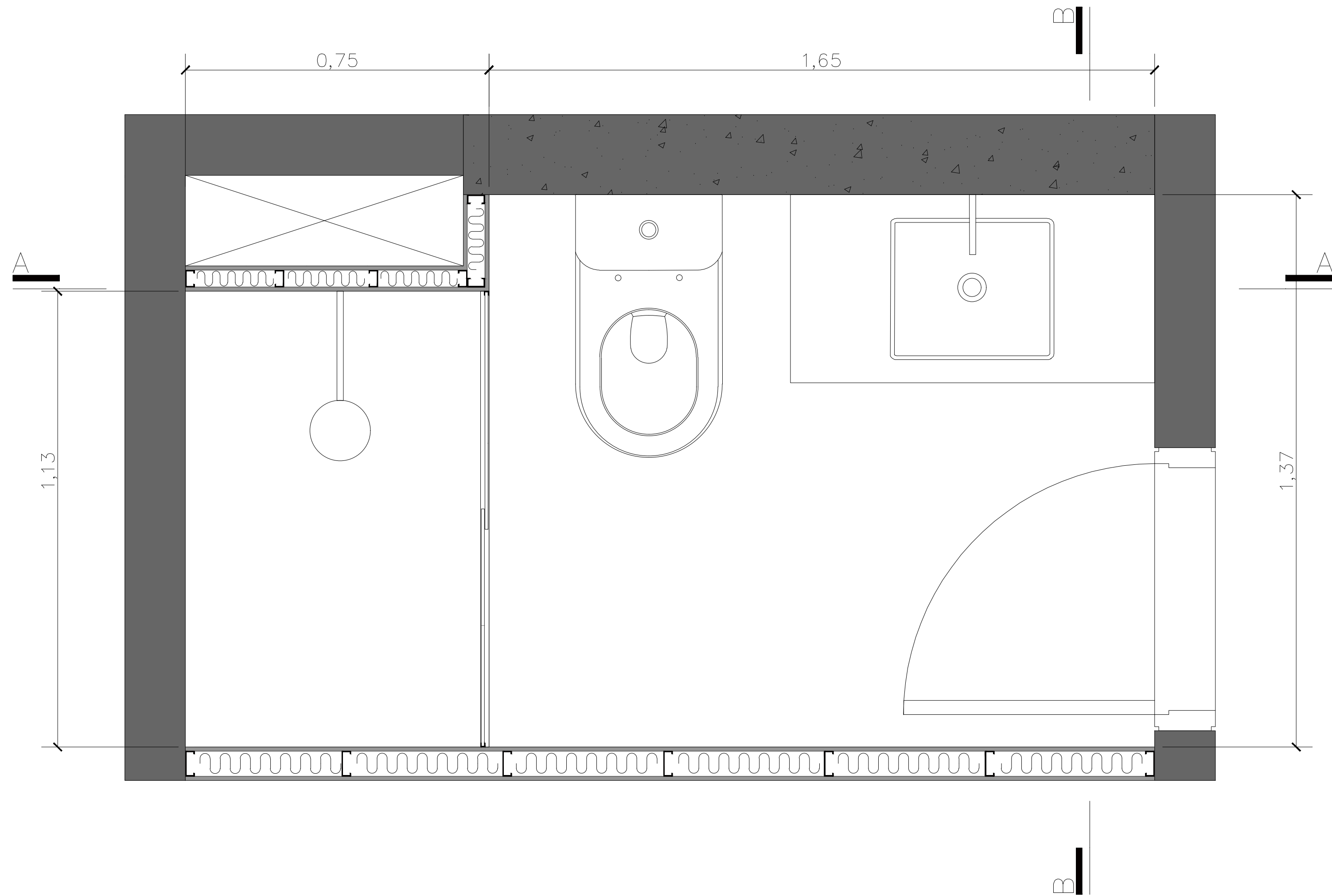
Planta Banheiro
