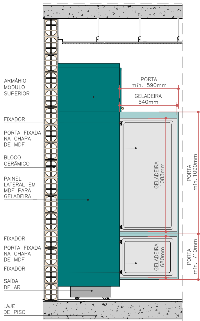
CORTE ESC. 1:25
