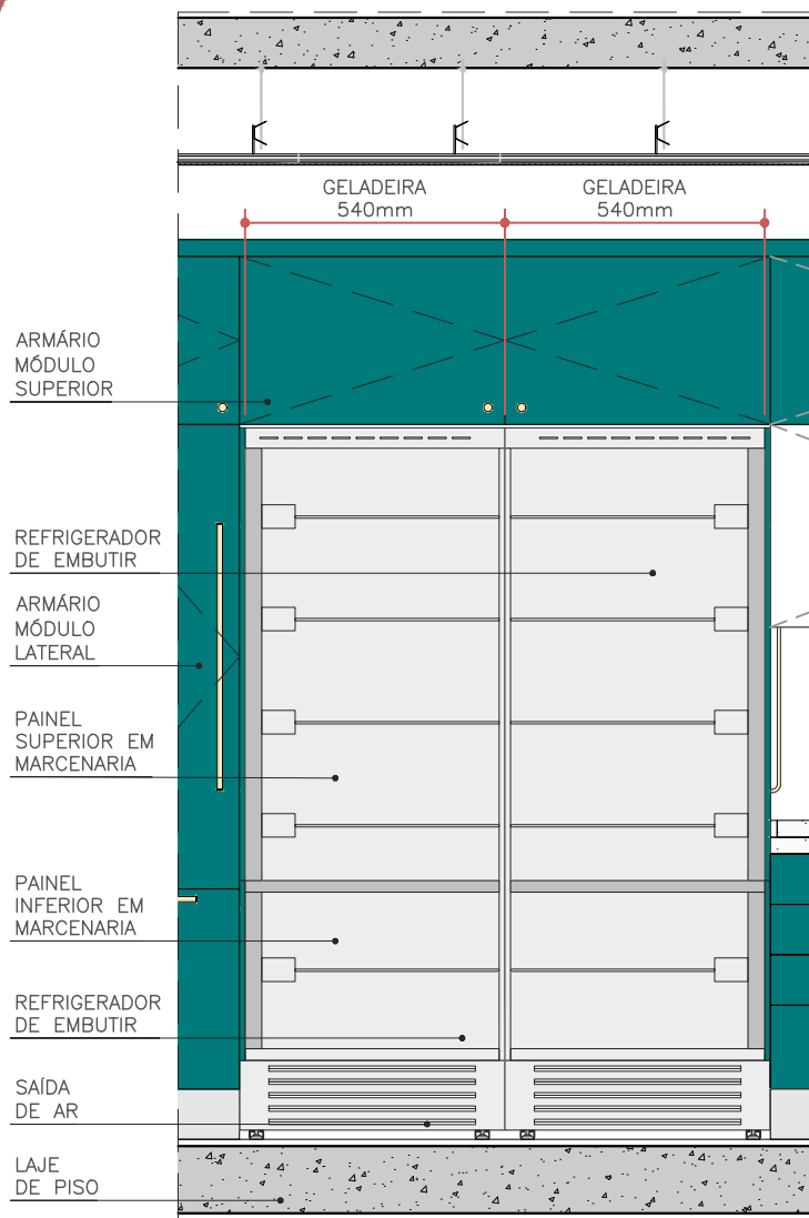
VISTA FRONTAL 02 ESC. 1:25
