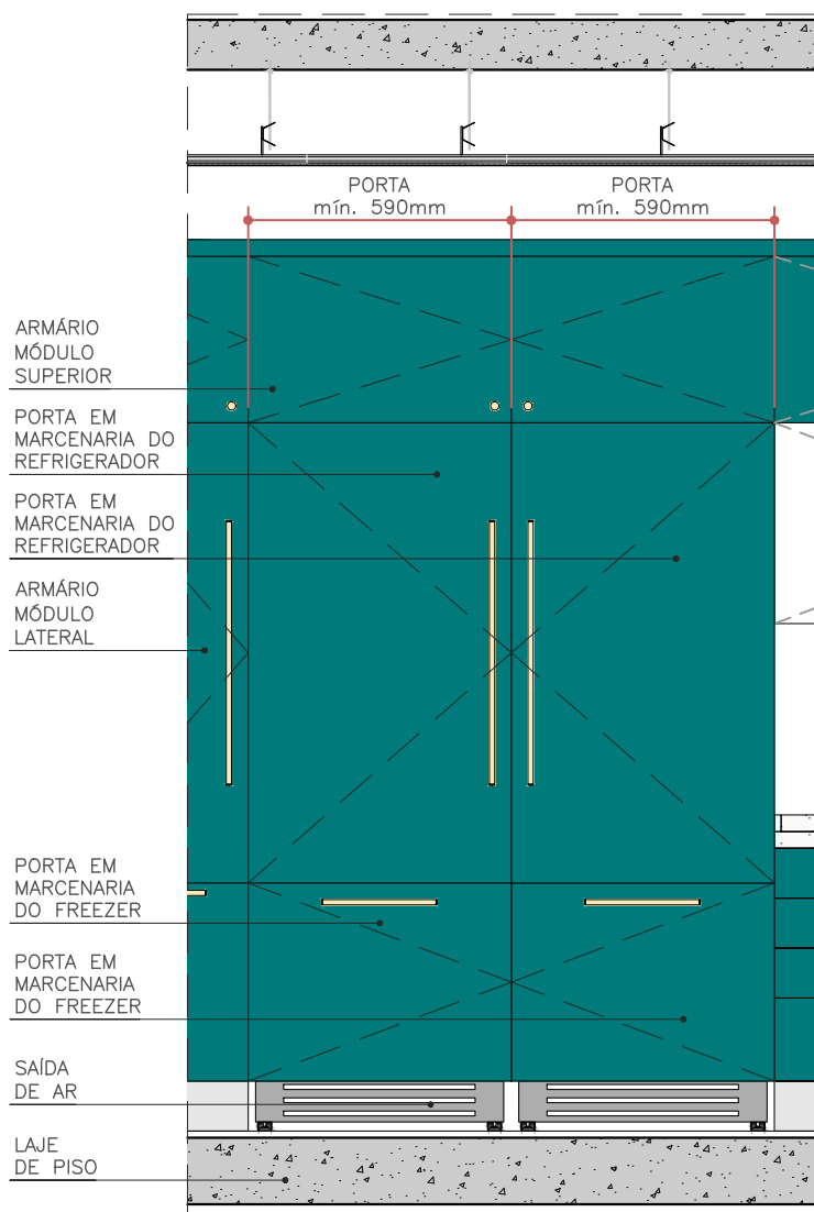
VISTA FRONTAL 01 ESC. 1:25
