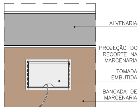
DET. PLANTA ESC. 1:10
