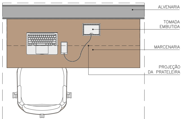
PLANTA ESC. 1:20
