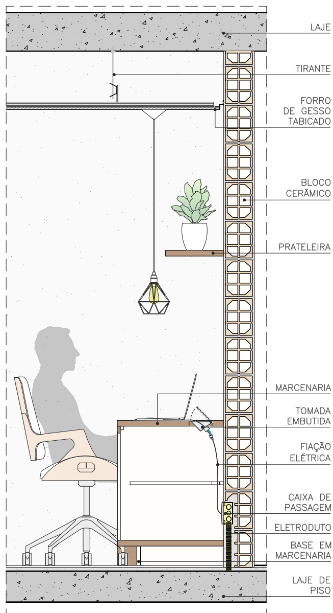
CORTE
