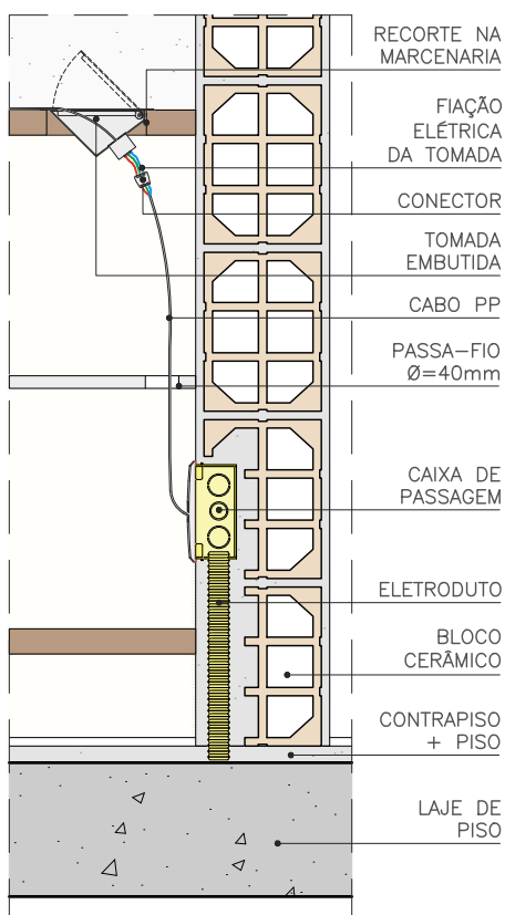
DET. CORTE ESC. 1:10
