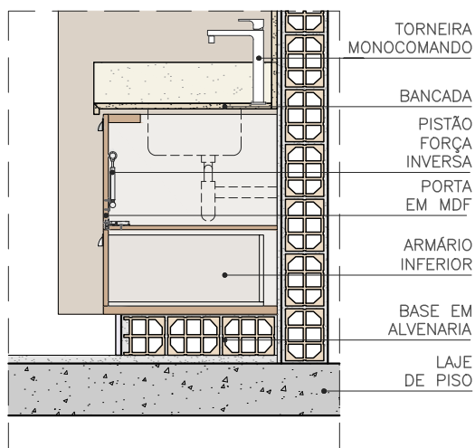
CORTE - PISTÃO ESC. 1:25
