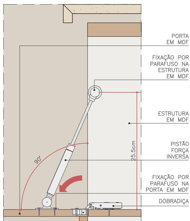
DET.2 PISTÃO ABERTO ESC. 1:5
