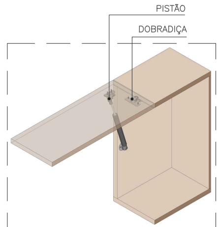
PISTÃO ABERTO SEM ESCALA
