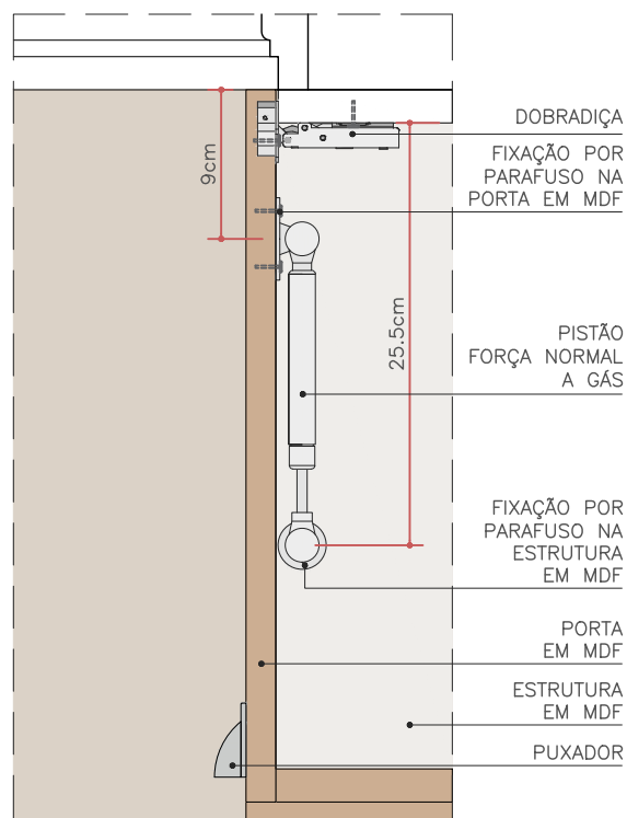
DET.1 PISTÃO FECHADO ESC. 1:5
