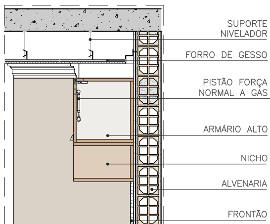
CORTE - PISTÃO ESC. 1:25
