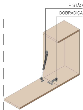
PISTÃO ABERTO SEM ESCALA
