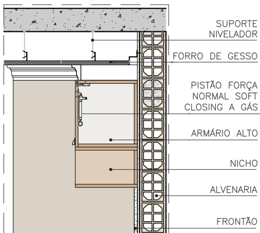
CORTE - PISTÃO ESC. 1:25
