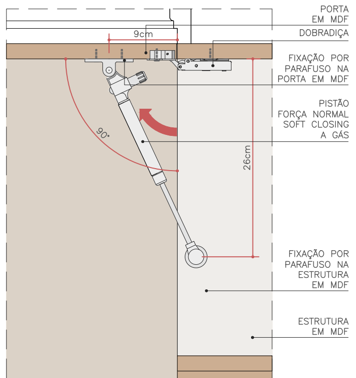
DET.2 PISTÃO ABERTO ESC. 1:5
