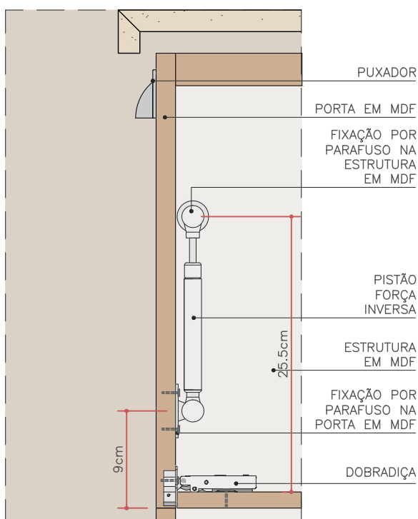
DET.1 PISTÃO FECHADO ESC. 1:5
