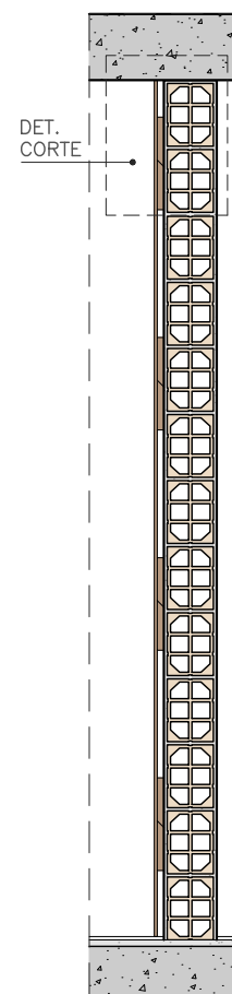
CORTE ESC. 1:25
