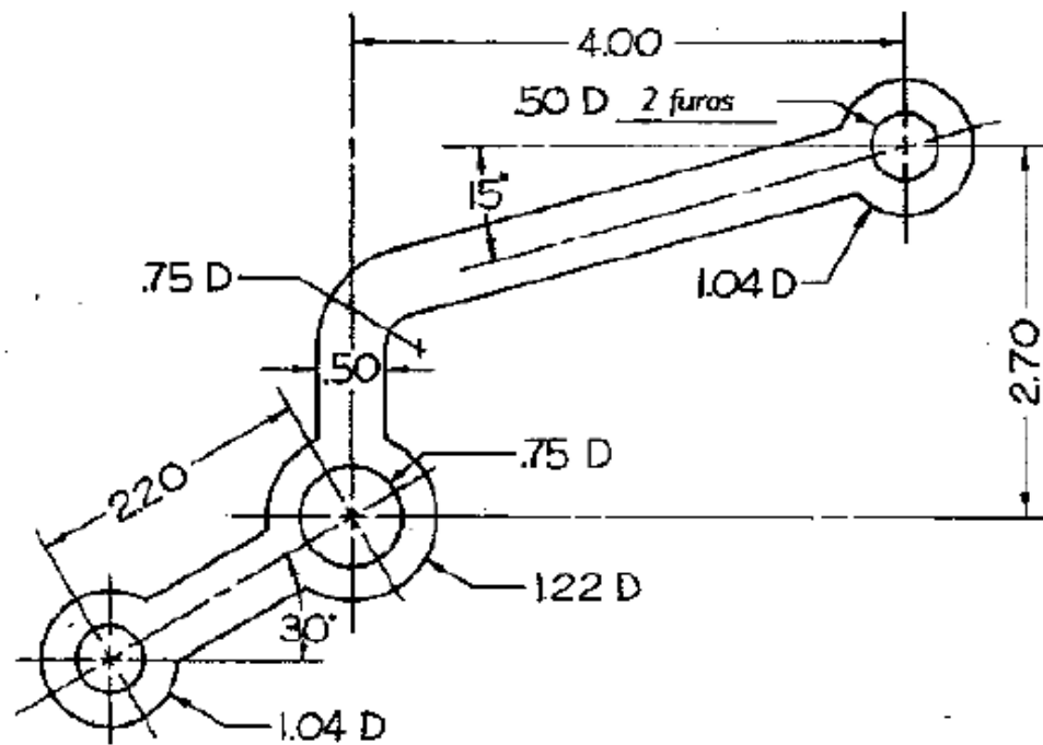
Cotovelo mecânico.
