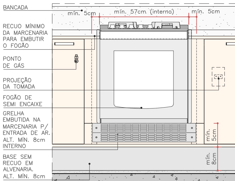
VISTA - GRELHA FRONTAL ESC. 1:15
