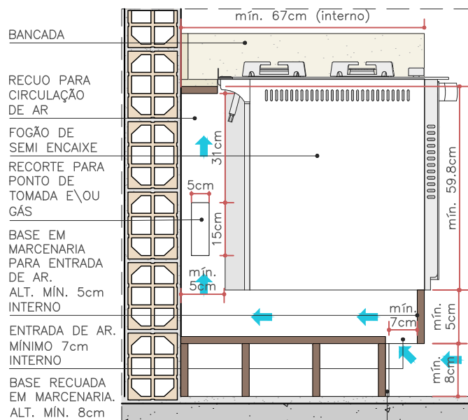
CORTE - BASE EM MARCENARIA ESC. 1:15
