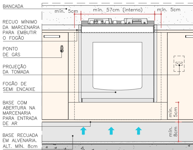
VISTA - BASE EM ALVENARIA ESC. 1:15
