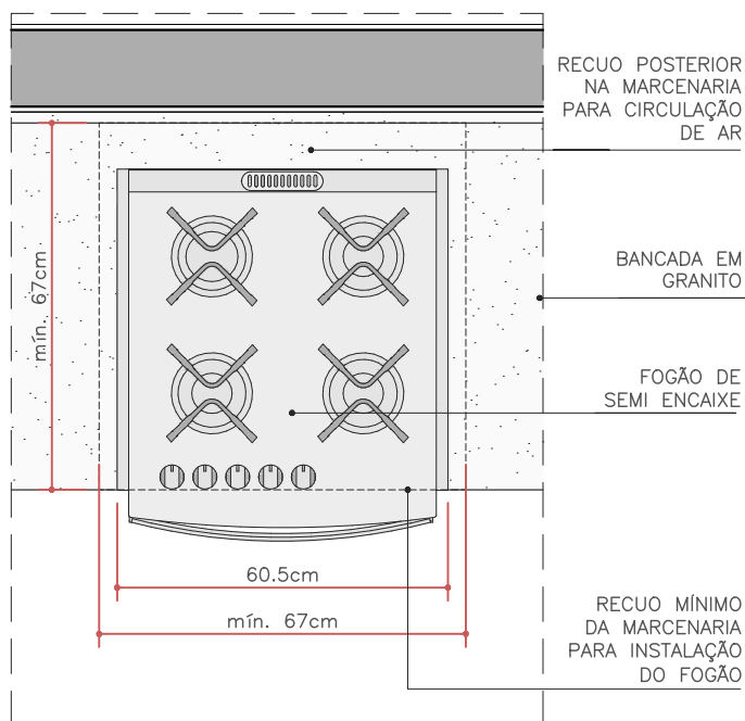
PLANTA ESC. 1:15
