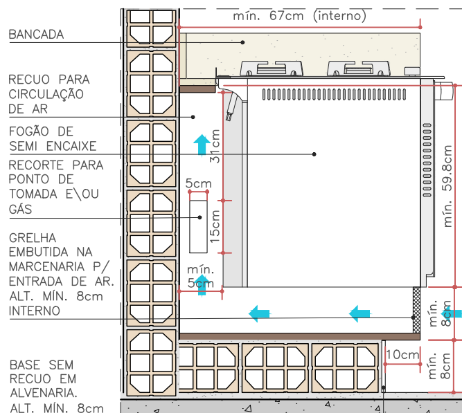
CORTE - GRELHA FRONTAL ESC. 1:15
