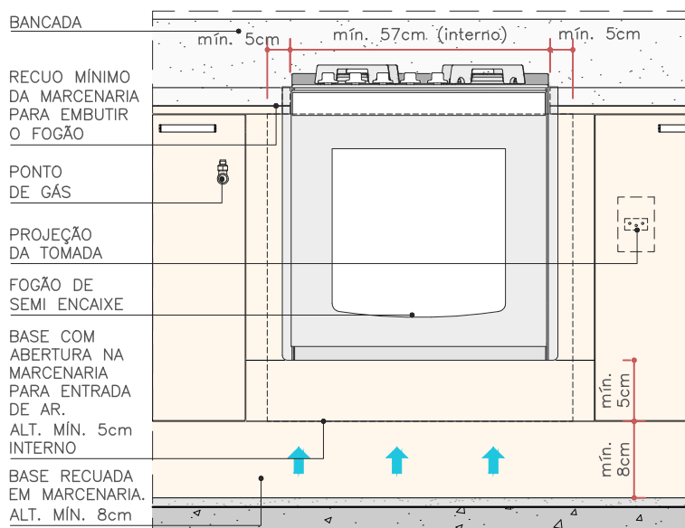
VISTA - BASE EM MARCENARIA ESC. 1:15
