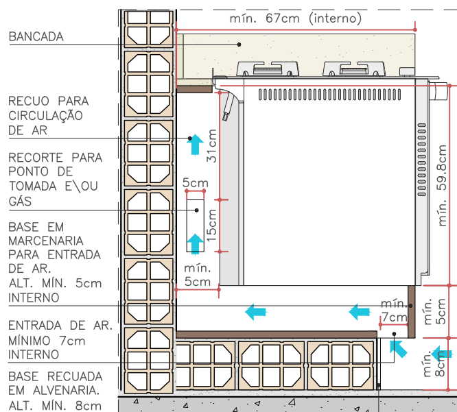
CORTE - BASE EM ALVENARIA ESC. 1:15
