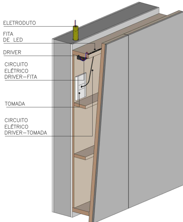
ISOMÉTRICA SEM ESCALA
