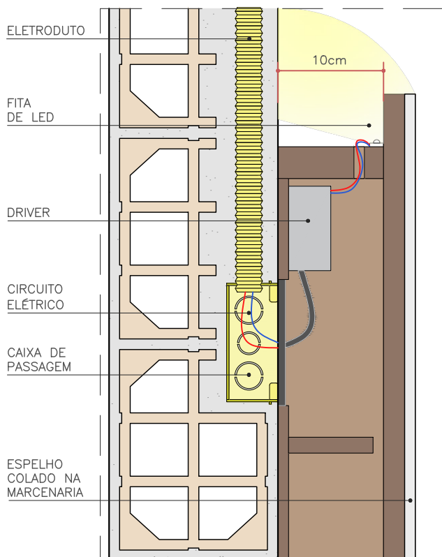
DET. COM CONEXÃO DIRETA ESC. 1:5
