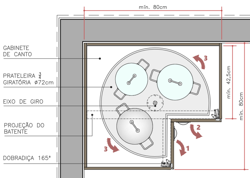
CANTO 3/4 - FECHADO ESC. 1:15
