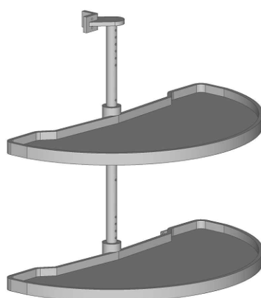
CANTO 1/2 LUA - ISOMÉTRICA 3 SEM ESCALA
