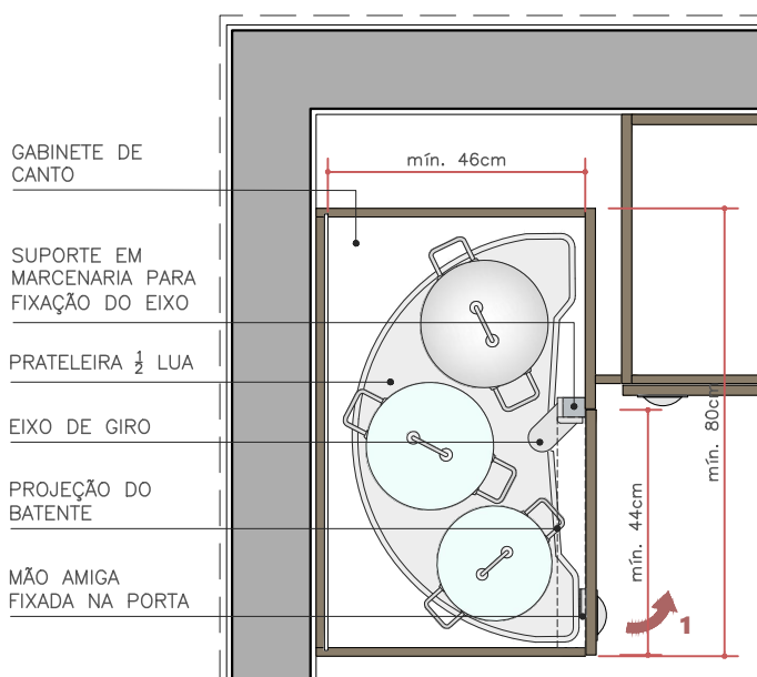
CANTO 1/2 LUA - FECHADO ESC. 1:15
