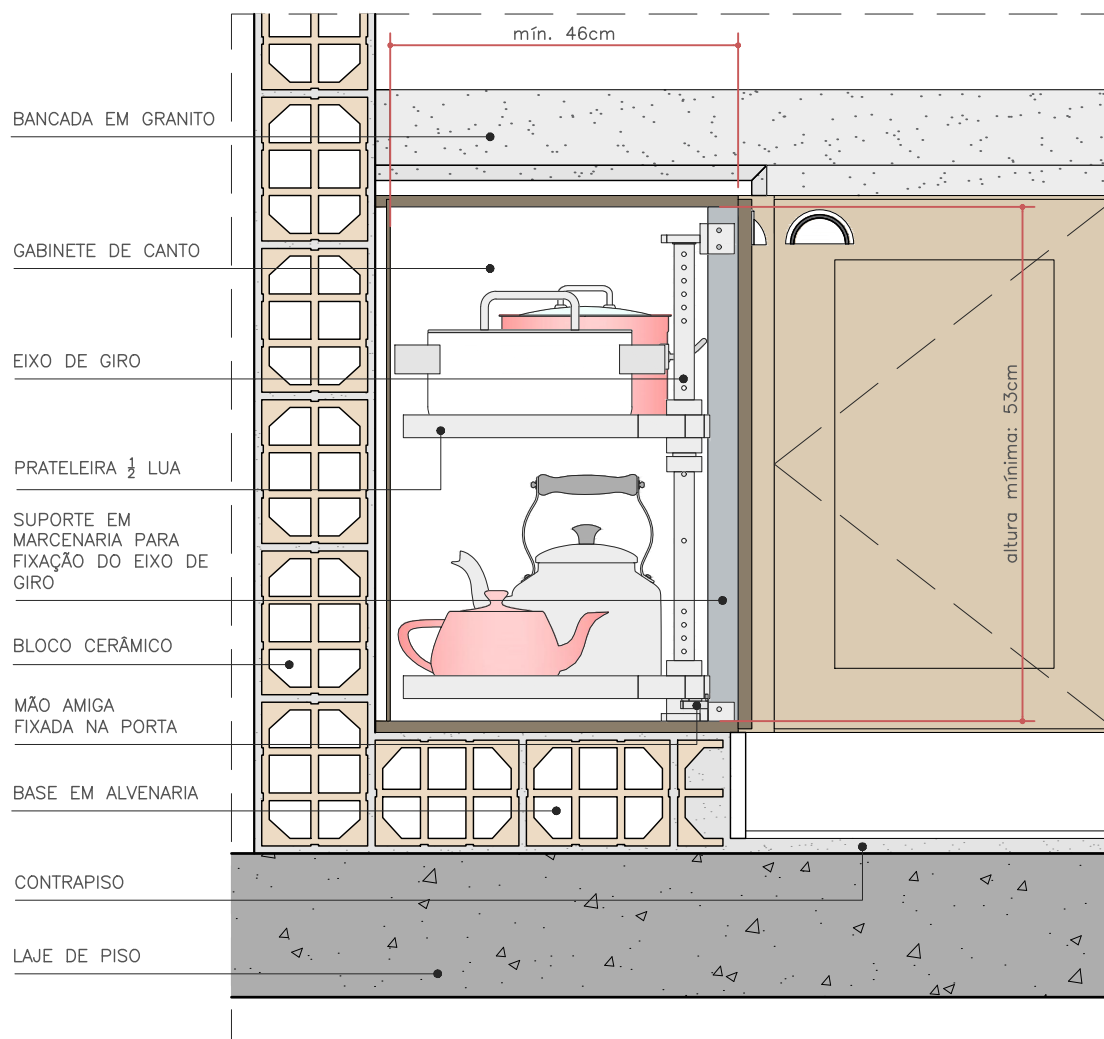
CANTO 1/2 LUA - CORTE ESC. 1:10
