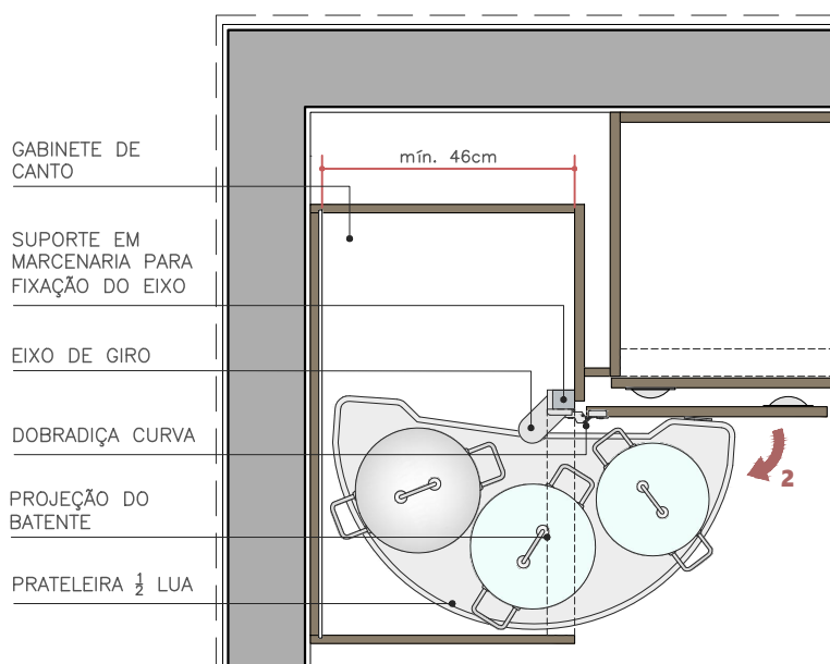
CANTO 1/2 LUA - ABERTO ESC. 1:15
