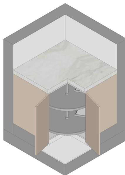
CANTO 3/4 - ISOMÉTRICA 2 SEM ESCALA
