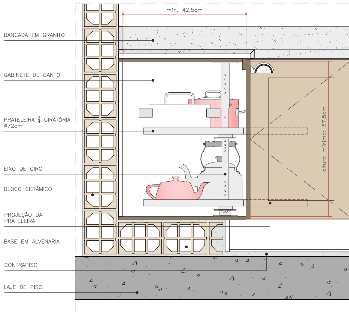
CANTO 3/4 - CORTE ESC. 1:10
