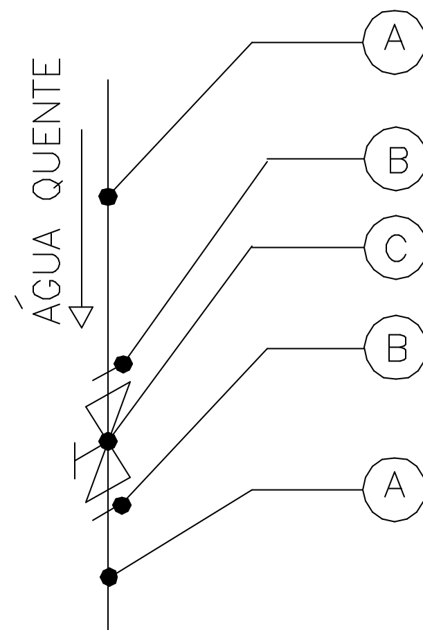
DETALHE DE INSTALAÇÃO DE REGISTRO DE GAVETA P/ ÁGUA QUENTE
