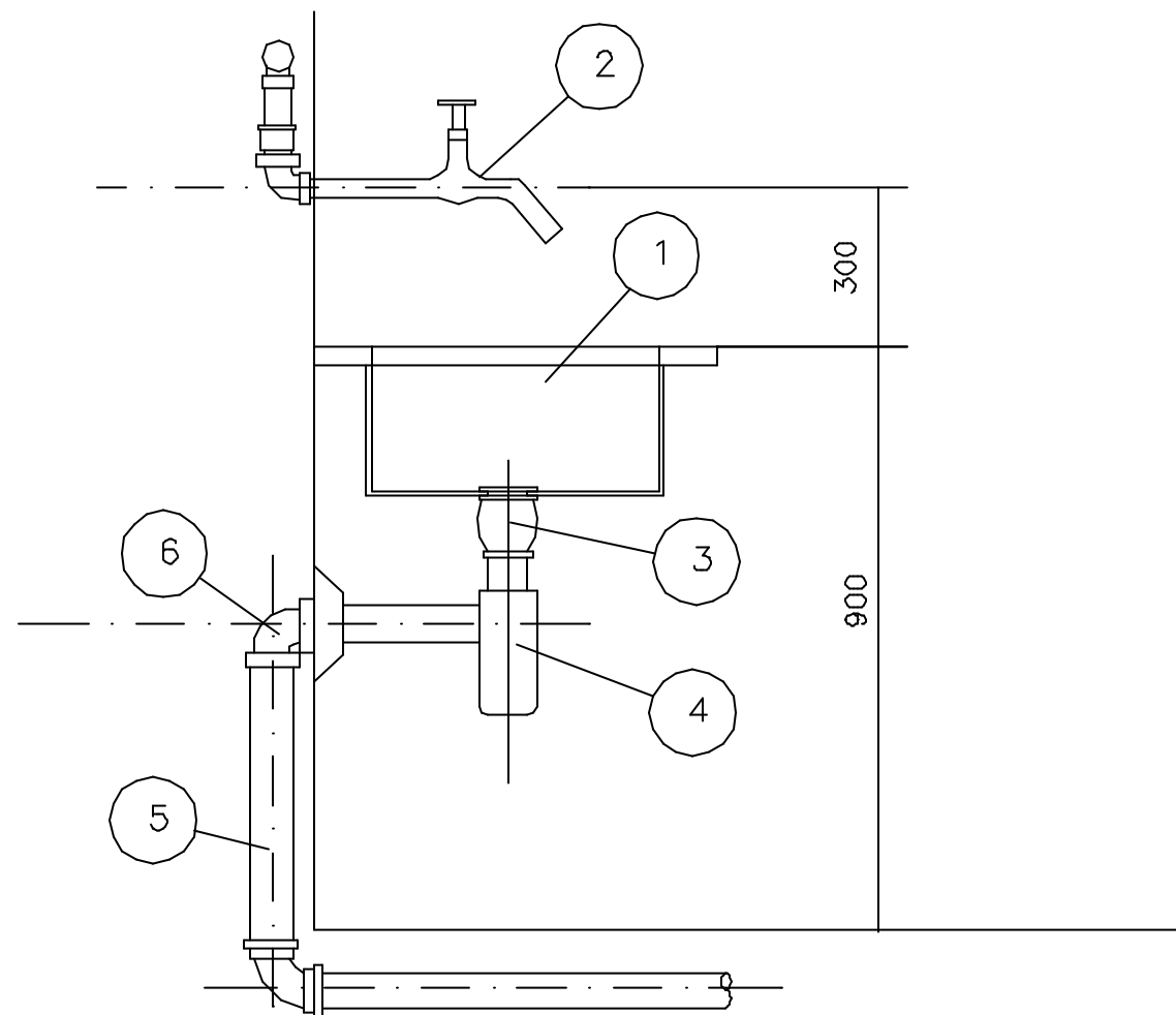
CORTE A-A
