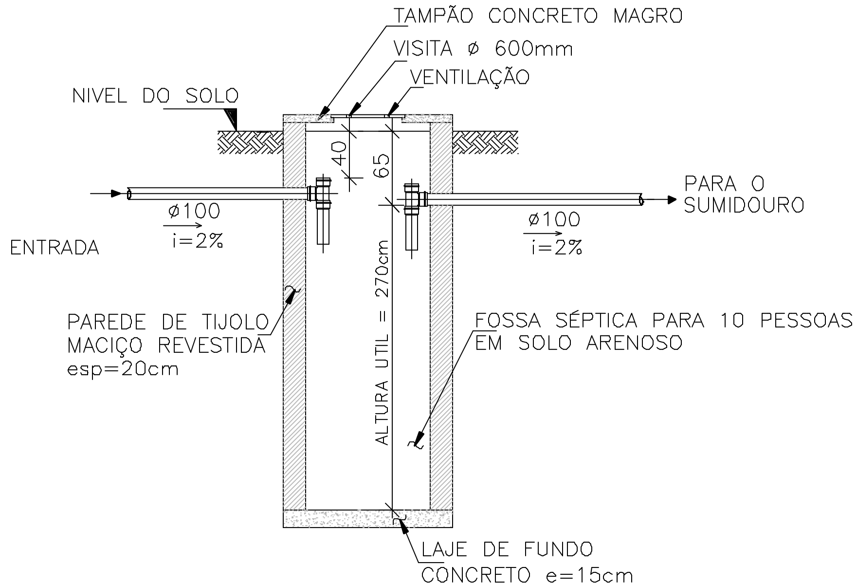
DETALHE DA FOSSA SÉPTICA
