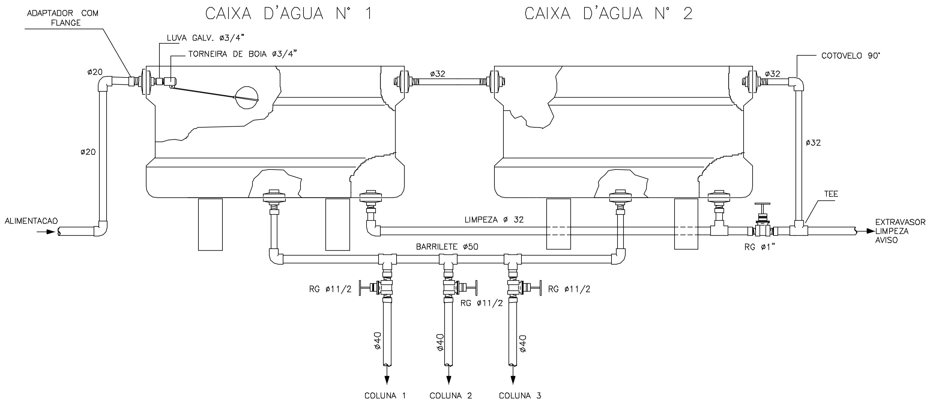
DETALHES DA LIGAÇÃO DAS CAIXAS D'AGUA
