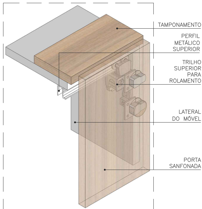
DET. TRILHO SUPERIOR FECHADO SEM ESCALA
