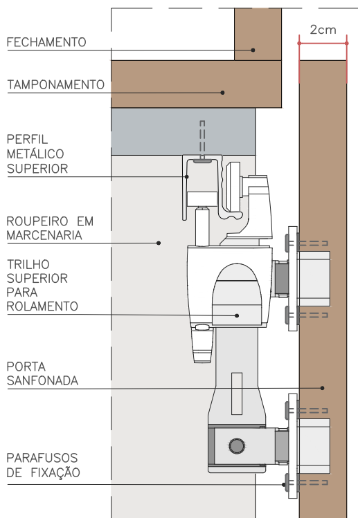
DET. TRILHO SUPERIOR FECHADO ESC. 1:2
