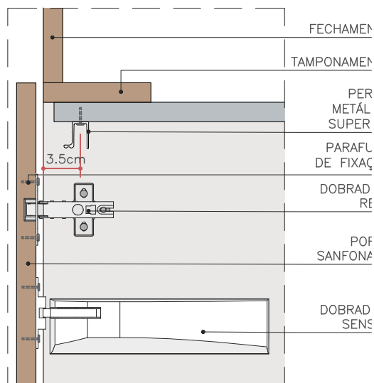
DET. DOBRADIÇA SENSYS FECHADA ESC. 1:5
