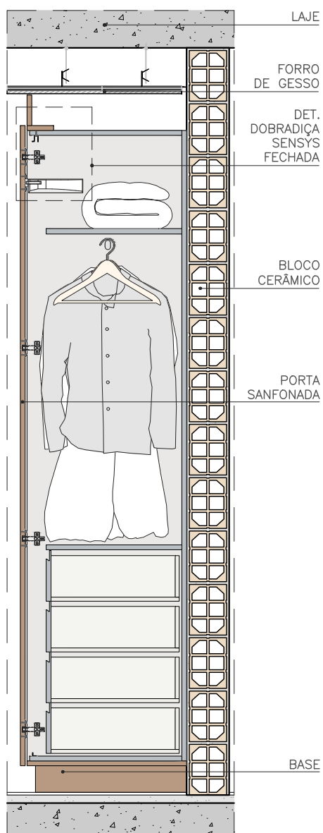
CORTE A - DOBRADIÇA SENSYS FECHADA ESC. 1:20
