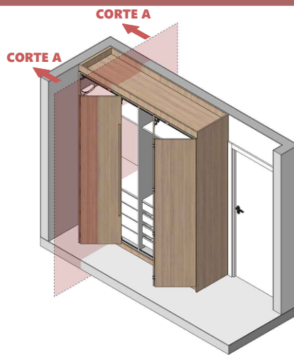
ISOMÉTRICA - MEIA ABERTURA SEM ESCALA
