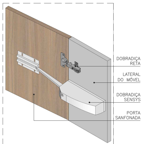
ISO - DET. DOBRADIÇA SENSYS ABERTA SEM ESCALA
