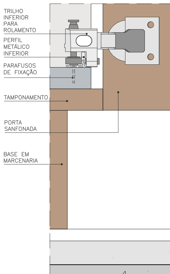
DET. TRILHO INFERIOR ABERTO ESC. 1:2
