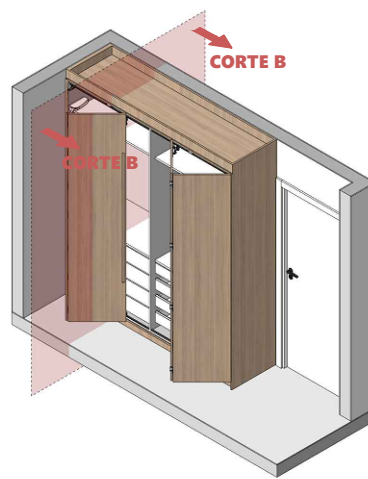
ISOMÉTRICA - MEIA ABERTURA SEM ESCALA
