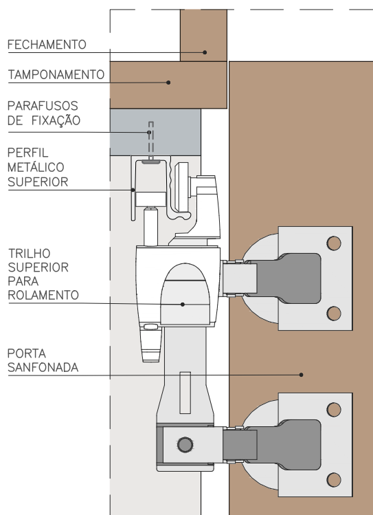
DET. TRILHO SUPERIOR ABERTO ESC. 1:2
