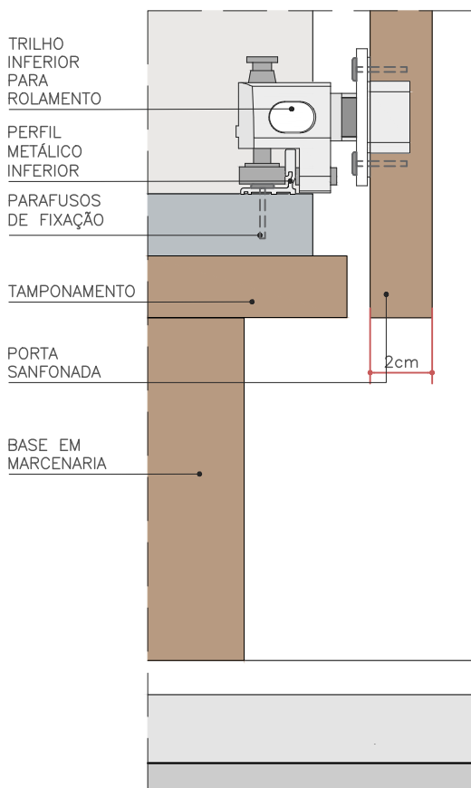
DET. TRILHO INFERIOR FECHADO ESC. 1:2
