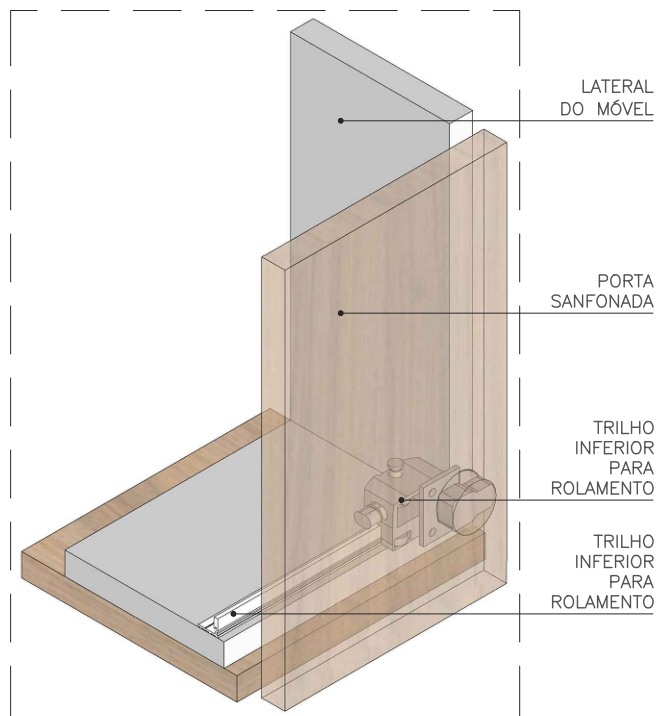
DET. TRILHO INFERIOR FECHADO SEM ESCALA
