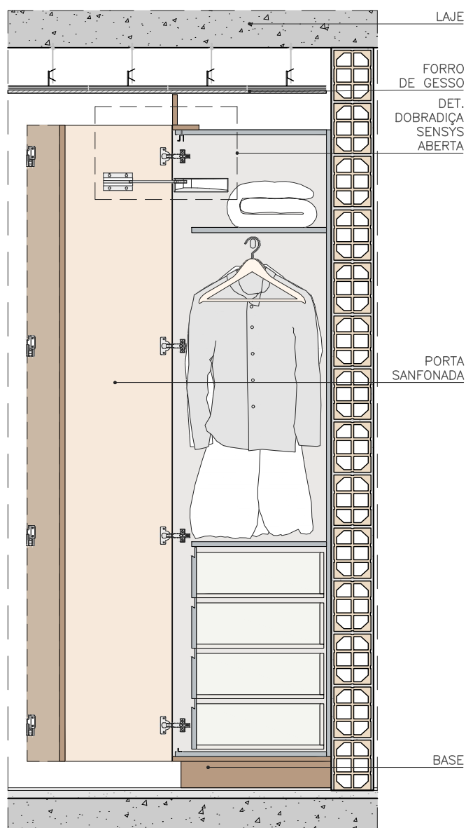
CORTE A - DOBRADIÇA SENSYS ABERTA ESC. 1:20
