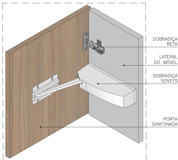
ISO - DET. DOBRADIÇA SENSYS FECHADA SEM ESCALA
