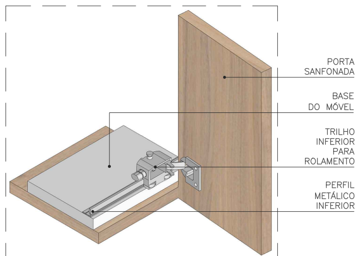
DET. TRILHO INFERIOR ABERTO SEM ESCALA
