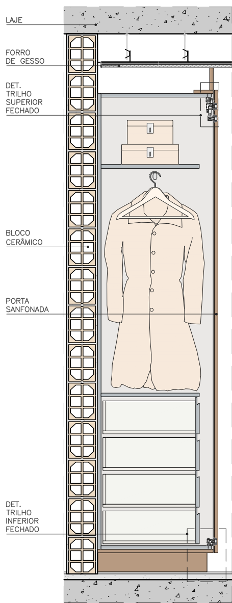
CORTE B - TRILHO FECHADO ESC. 1:20
