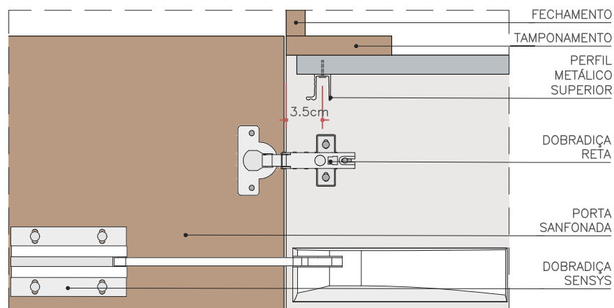
DET. DOBRADIÇA SENSYS ABERTA ESC. 1:5
