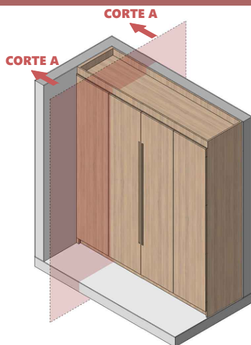
ISOMÉTRICA - FECHADO SEM ESCALA
