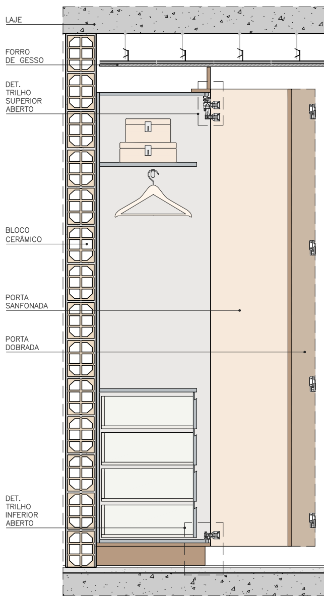
CORTE B - TRILHO ABERTO ESC. 1:20
