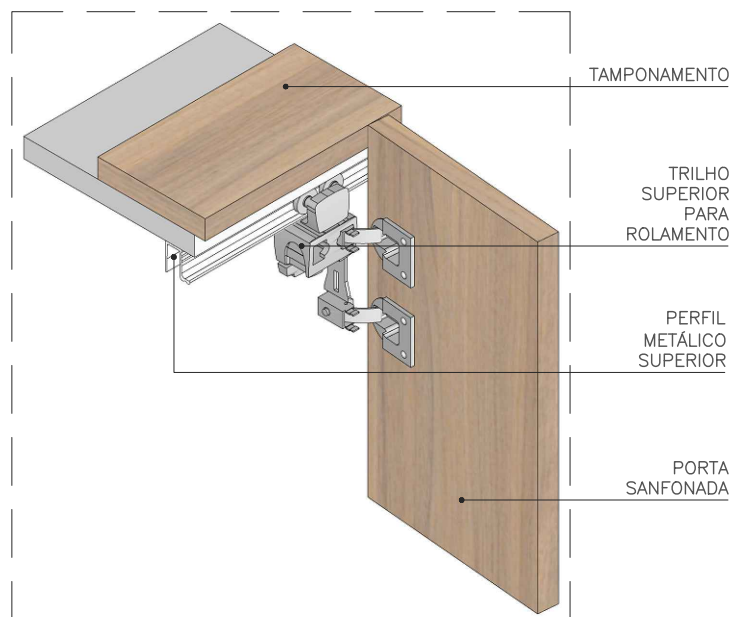
DET. TRILHO SUPERIOR ABERTO SEM ESCALA
