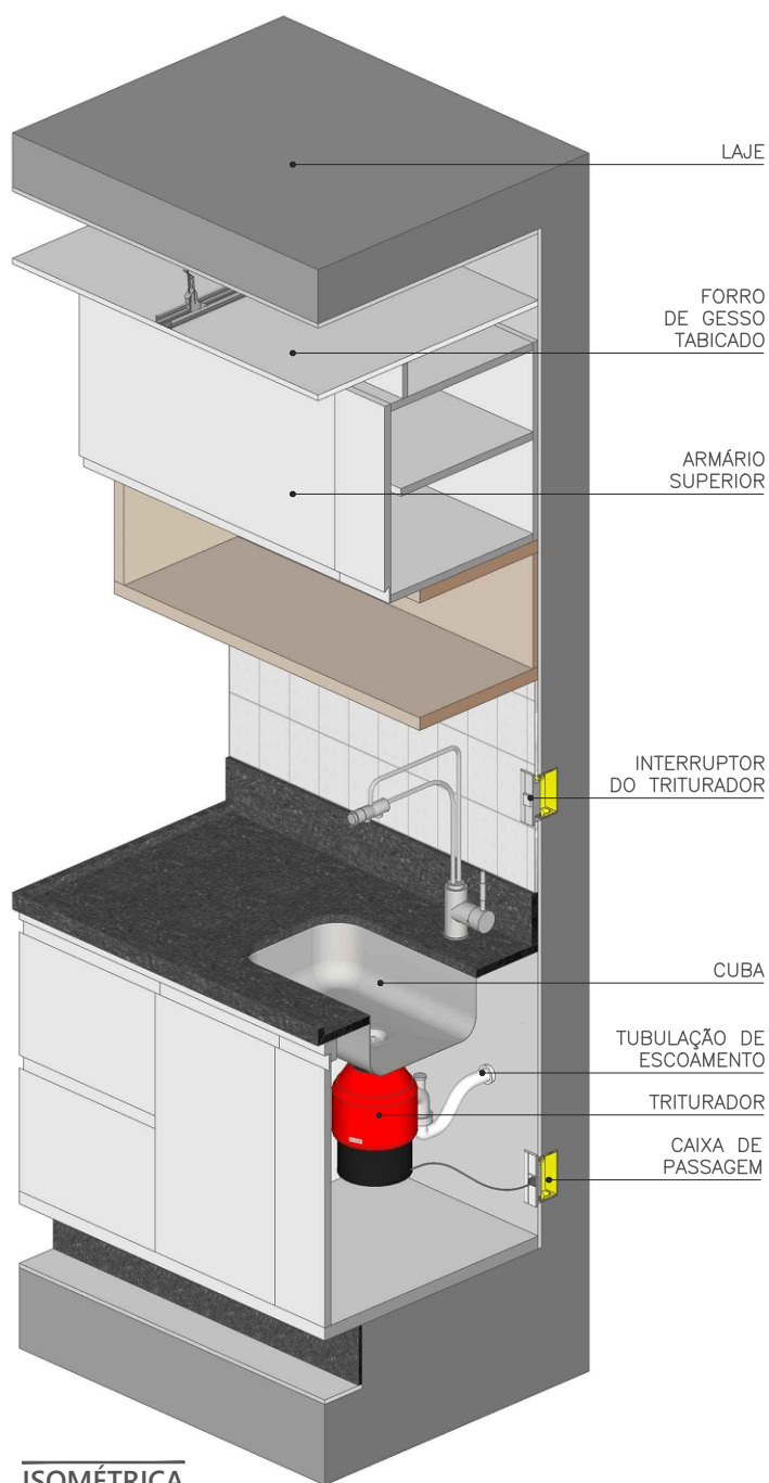
ISOMÉTRICA SEM ESCALA
