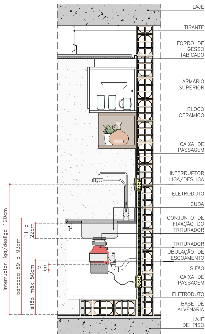
CORTE ESC. 1:20
