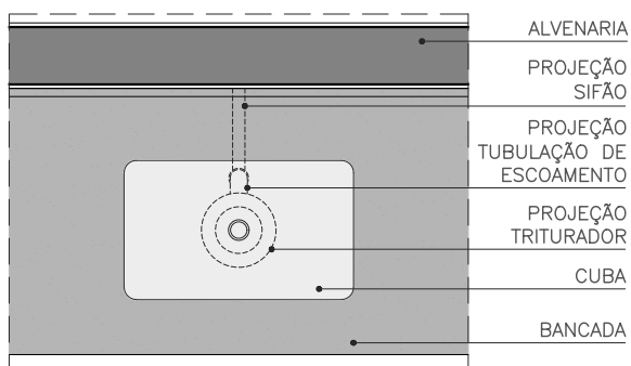
PLANTA ESC. 1:20
