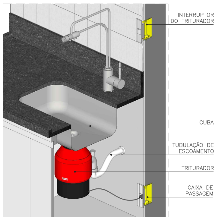
ISOMÉTRICA - DET. CORTE SEM ESCALA
