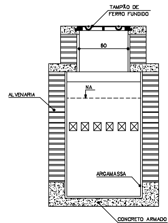
CORTE 2-2
