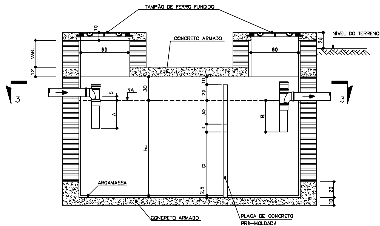
CORTE 1-1
