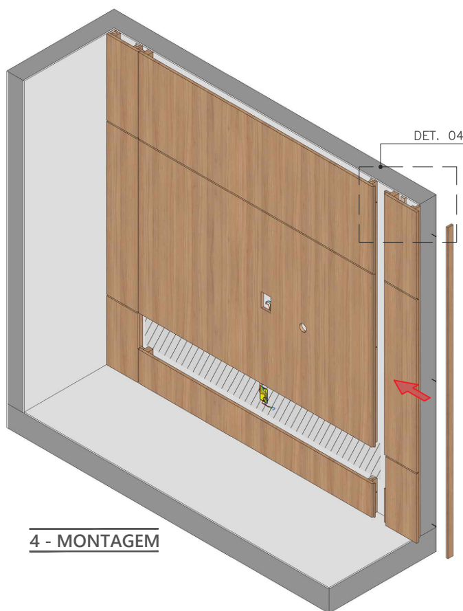
DET. 04 - MONTAGEM
