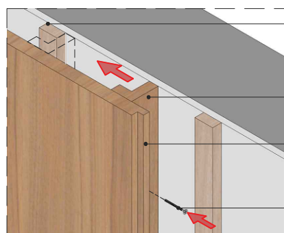
DET. 03 - MONTAGEM
