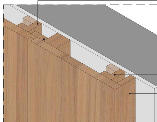
DET. 06 - PAINEL INSTALADO
