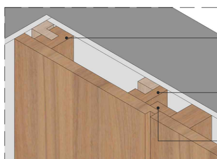
DET. 05 - PAINEL INSTALADO
