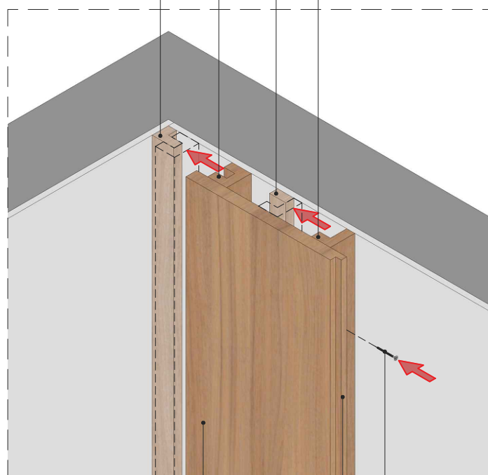
DET. 01 - MONTAGEM
