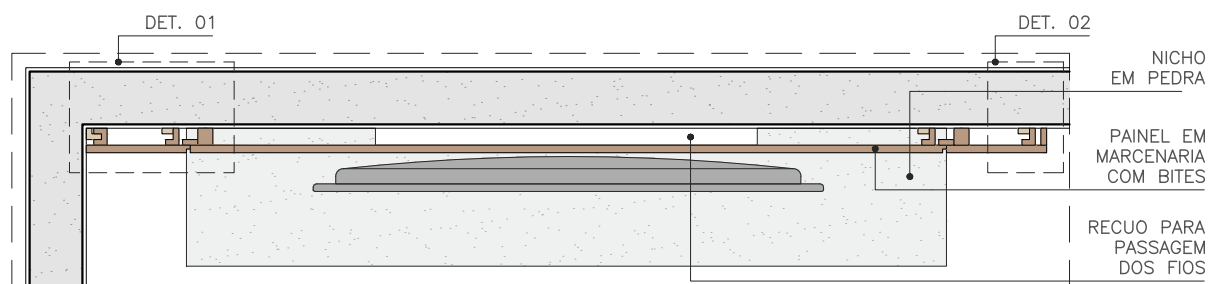
PLANTA ESC. 1:20
