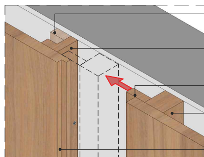
DET. 02 - MONTAGEM
