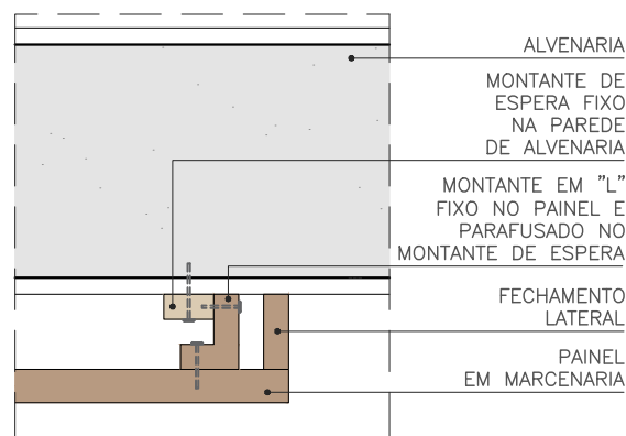
DET. 02 - PLANTA ESC. 1:5
