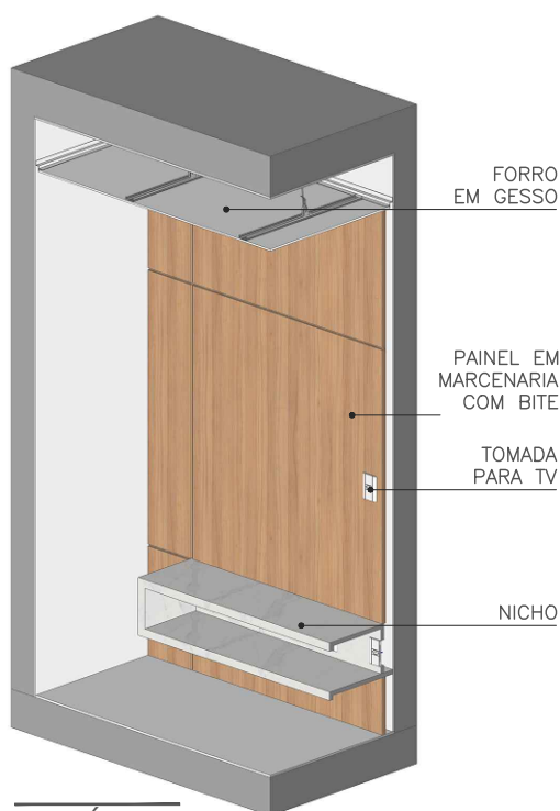
ISOMÉTRICA SEM ESCALA
