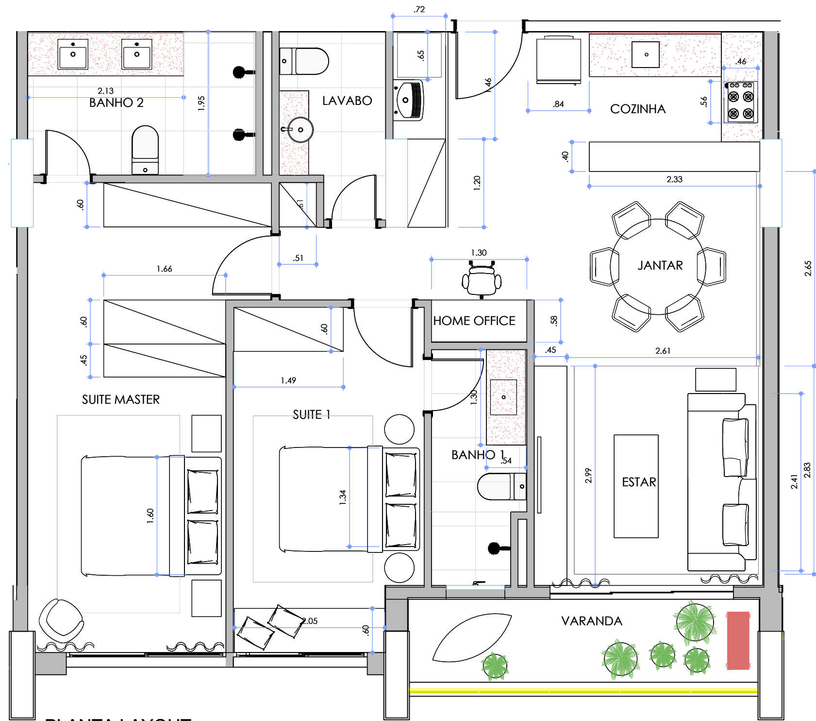
PLANTA LAYOUT DECORADO 80m2 ESCALA 1:50
