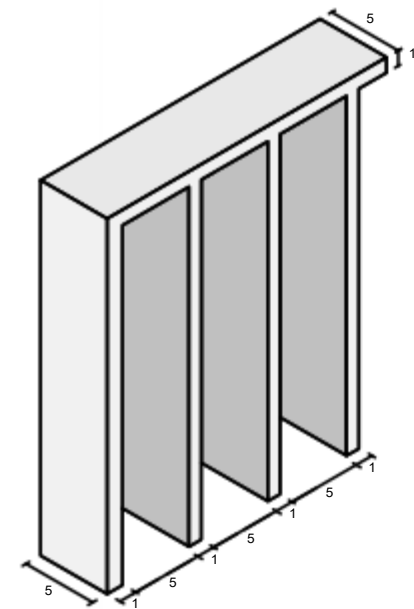
DETALHE GRADIL METÁLICO SEM ESCALA
